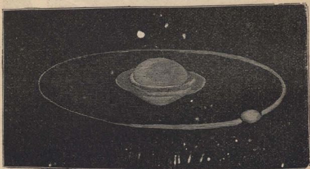
Formación i evol del planeta Saturno.
